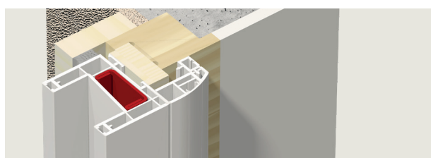
Profil compensateur pour tapées persiennes
