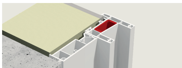
Tapées rapportées de 27,5 à 145 mm sans délignage
