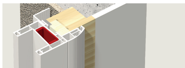
Dormant rénovation à fixation frontale
