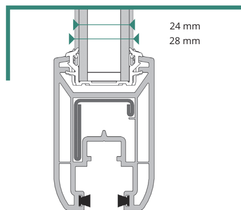
Remplissage de 24 ou 28mm
