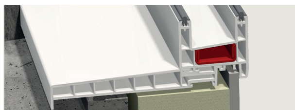
Pièces d'appui frontales ou par le dessous
